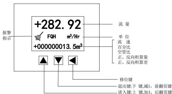
图 4.1 a 方表键盘定义与液晶显示
