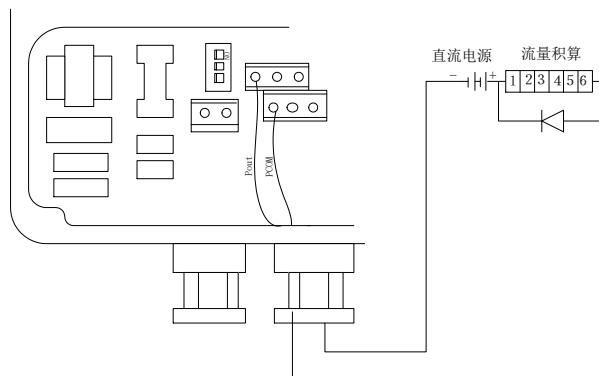
图 4.4 (b) 电磁计数器接线
