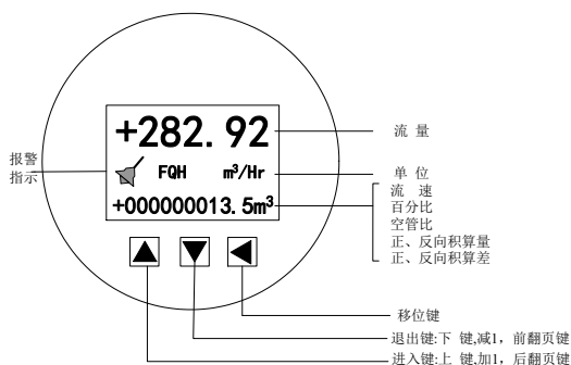
图 4.1 b 圆表键盘定义与液晶显示
