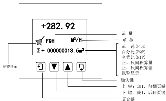
图 4.1 c 方表键盘定义与液晶显示
