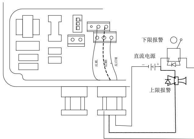
图 4.4 (d) 报警输出接线
