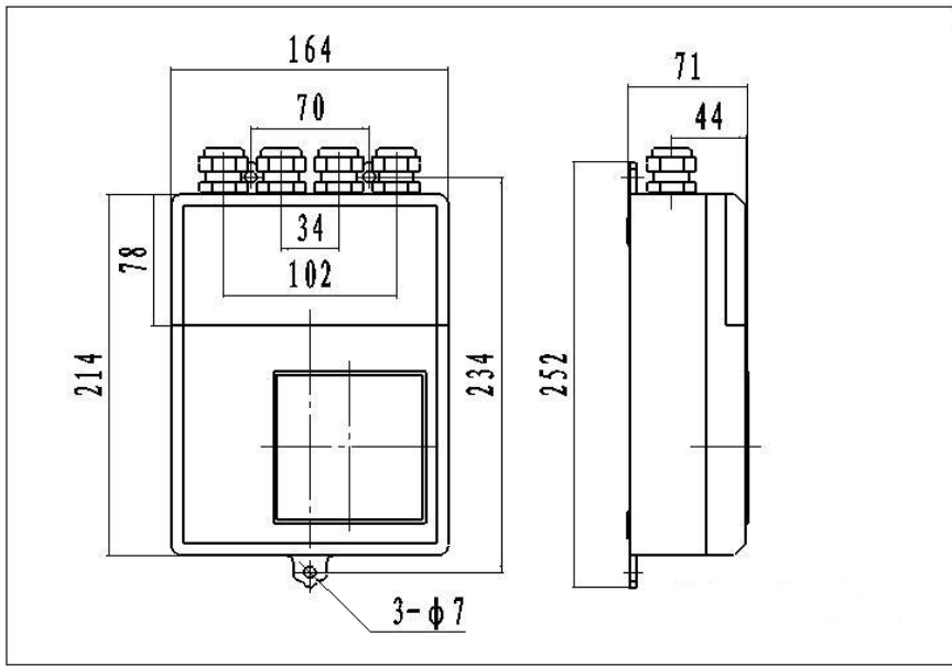
图 3 方型壳体分体式外型尺寸图
