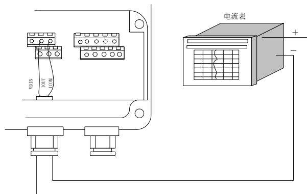
图 4.4 (a) 电流输出接线图
