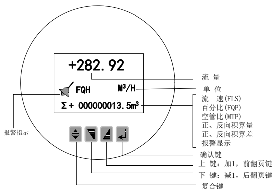
图 4.1 d 圆表键盘定义与液晶显示
