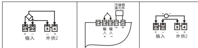
(7) 仪表与3线制电压、电流变送器的接线
